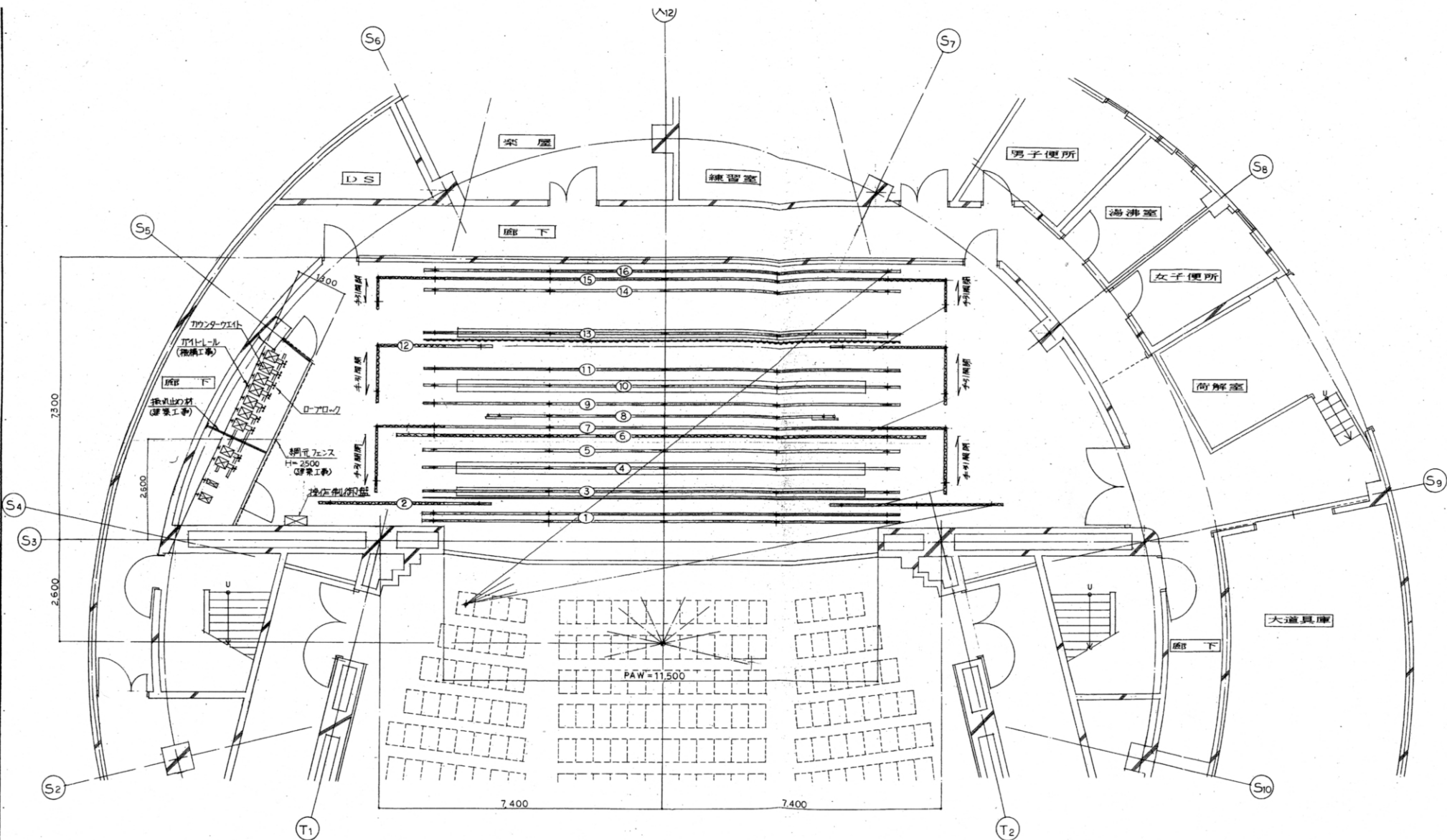
舞台平面配置図 1/50
